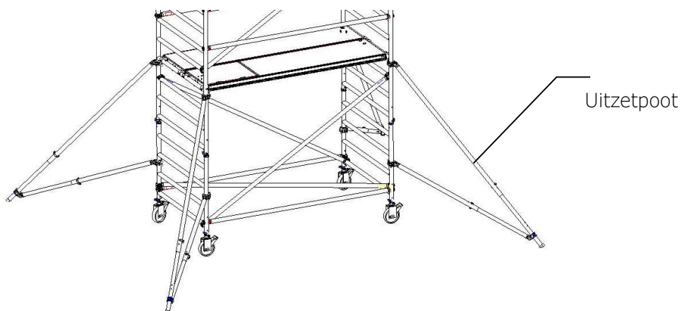
Rolsteiger met uitzetbogen
