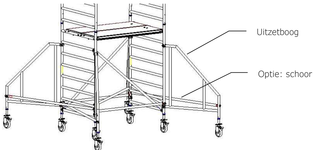
Rolsteiger met uitzetbogen
